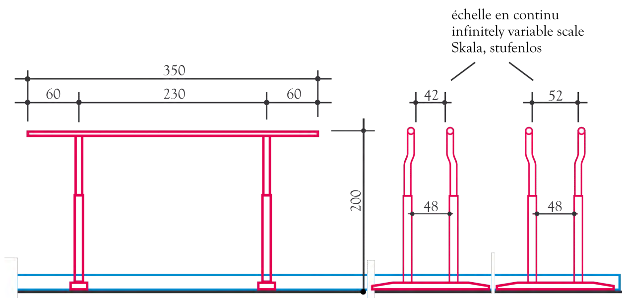
vue de côté side view Ansicht Längsseite
