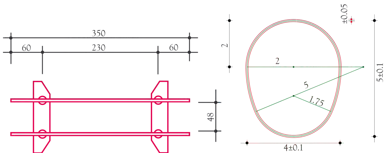
vue de dessus top view Aufsicht
