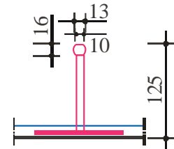
vue de face front view Ansicht Stirnseite
